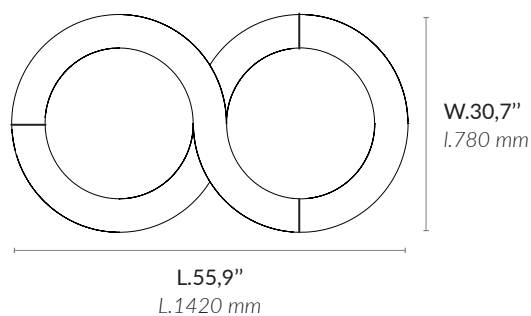
Bottom view Vue de dessous
